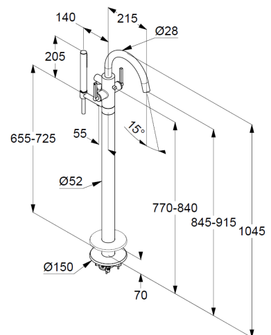
Maßzeichnung
