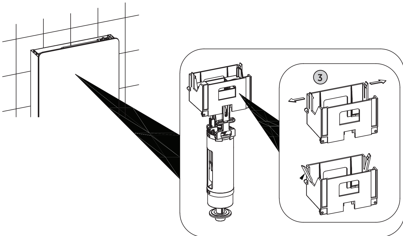
Verschlüsse an der Befestigungseinheit Buckles on the cistern hanging plate
