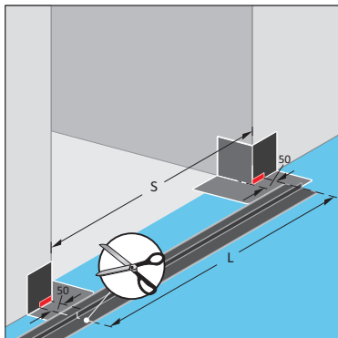
G1.3. Kapillarschutzband ablängen auf: lichtes Maß S + 2 \times 50 mm.
