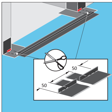
G1.4. Kapillarschutzband rechts und links 50 mm zum Durchgang ausklinken.
