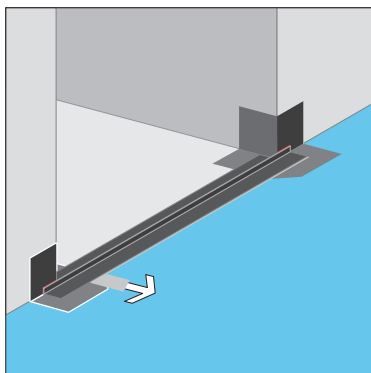
G1.5. Schutzfolien rückseitig abziehen und das Kapillarschutzband mit den beiden Außenecken und am Boden verbinden.
