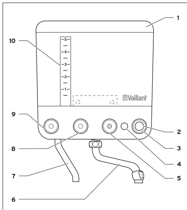
Abb. 3.1 Bedienelemente
