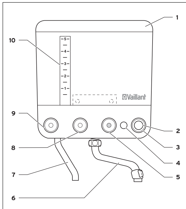
Fig. 3.1 Panneau de commande
