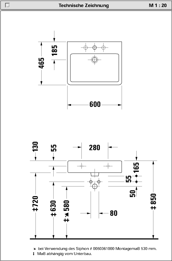
Vero Waschtisch # 0454600000/# 0454600030/# 0454600060 ↔ 600 mm ↔
