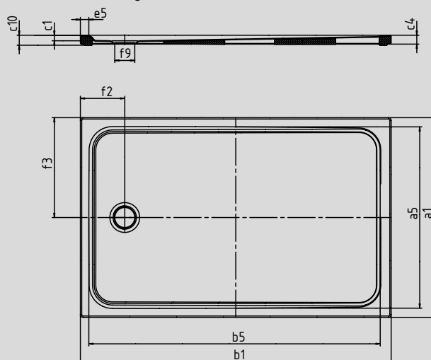
Modell 2266 mit Wannenträger extraflach
