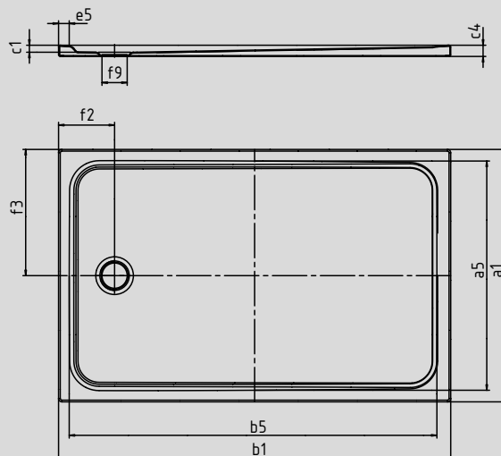
Modell 2266 mit Wannenträger extraflach
