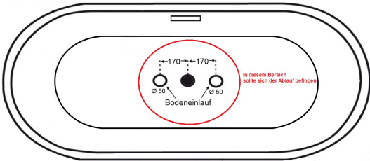
Montage des Wannenablaufs
