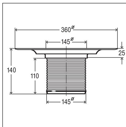
Abb. 4: Maßzeichnung für Modell 4994
