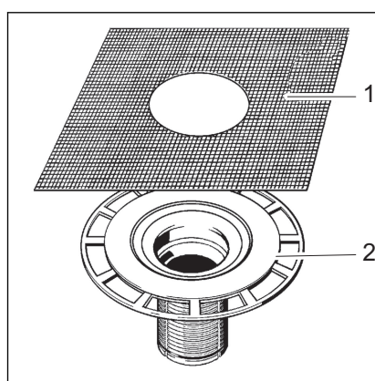
Abb. 1: Bauteile Aufstockelement Modell 4994
