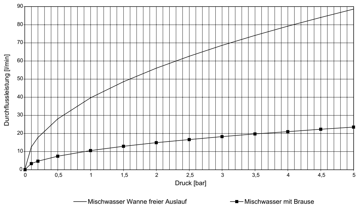
Bade-4-Locharmatur mit Schwallauslauf gültig für die Linien Ceratop, Dallas
