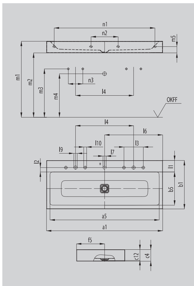
Drehknopfbohrungen für Ab- und Überlaufventil CLOU mit Kabelzug und Drehknopf
