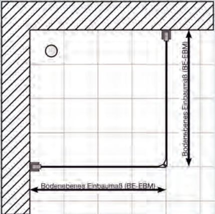
Montage Bodeneben
