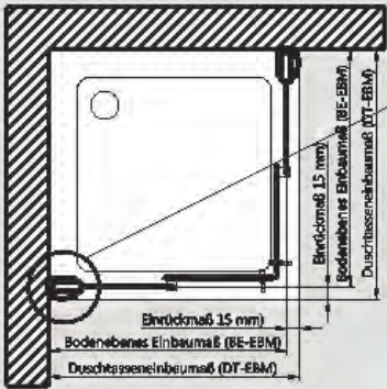
Montage auf Duschtasse
