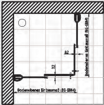
Montage Bodeneben
