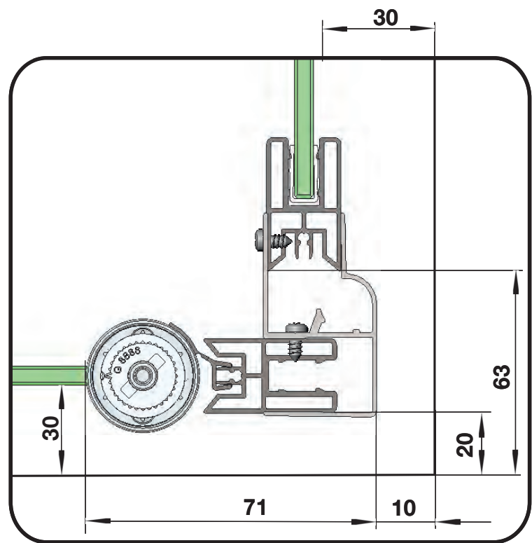
Montage Bodeneben
