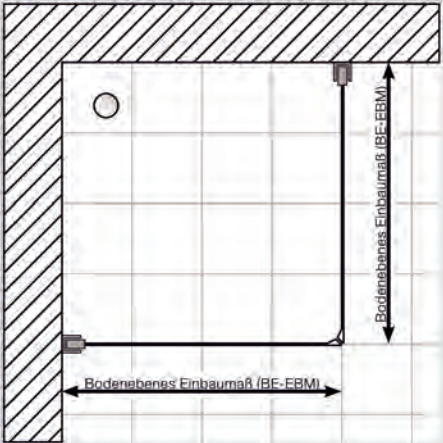
Montage Bodeneben
