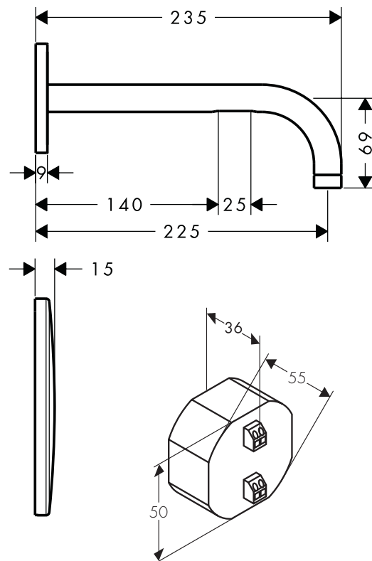
AXOR Uno 38120XXX
