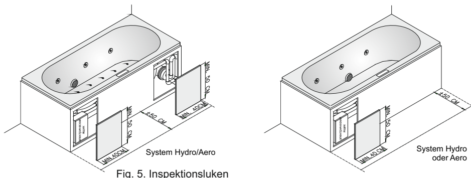
Fig. 5. Inspektionsluken
