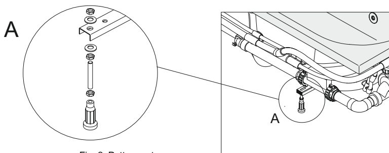
Fig. 2 Patte montage
