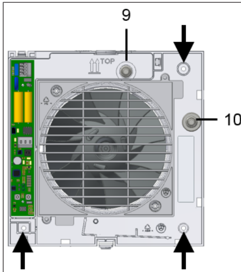
9 Leitungstülle
