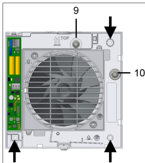
9 Cable grommet
