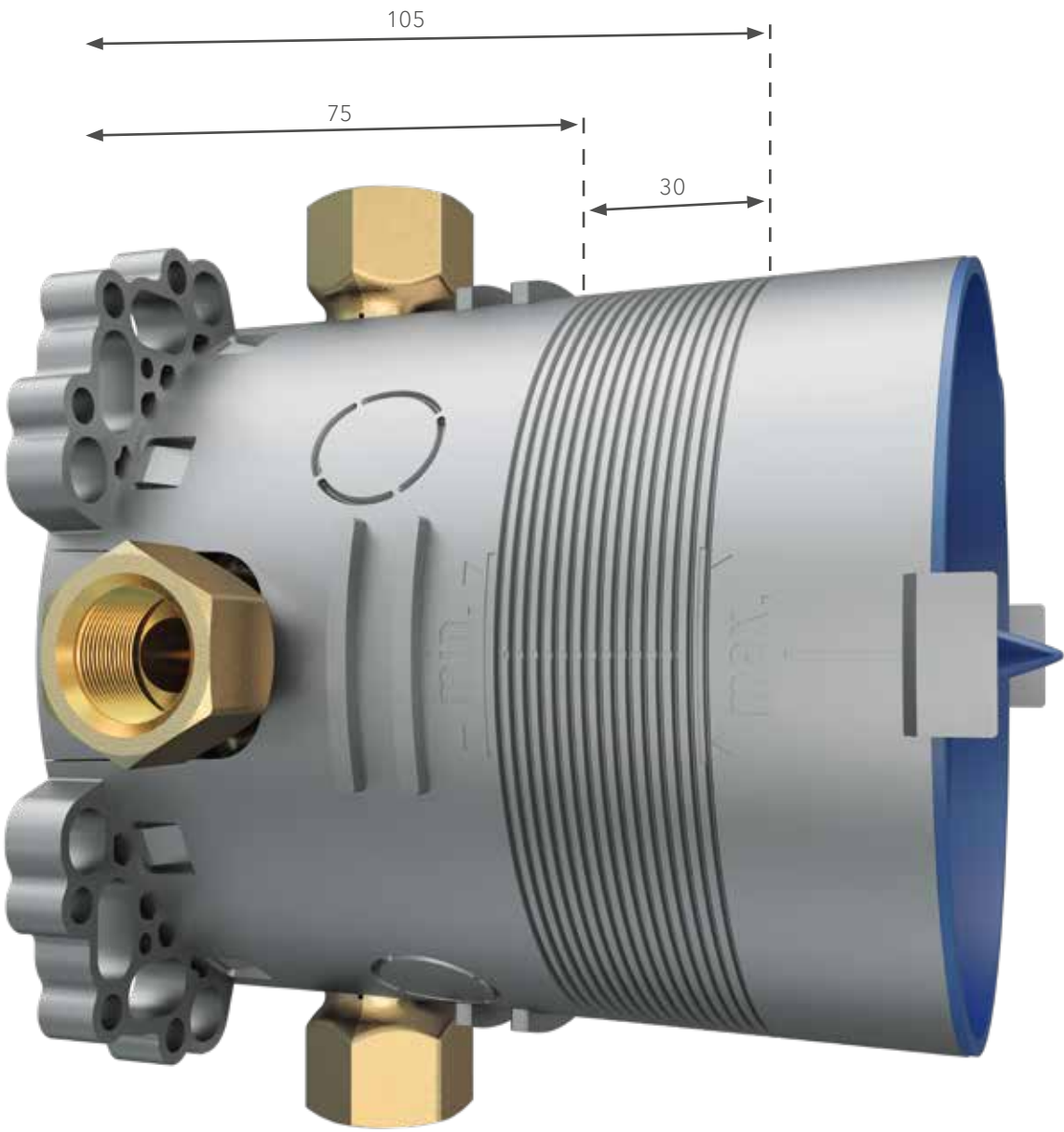
Höchste Ingenieurskunst: Die HANSABLUEBOX-Universal-Grundeinheit bietet komfortable 31 mm Abstand vom Anschluss zur Wand und einen breiten Spielraum von 75 – 105 mm bei der Einbautiefe.
