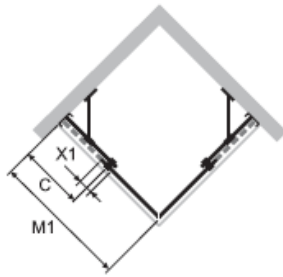
Linksbefestigung
