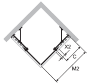
Rechtsbefestigung
