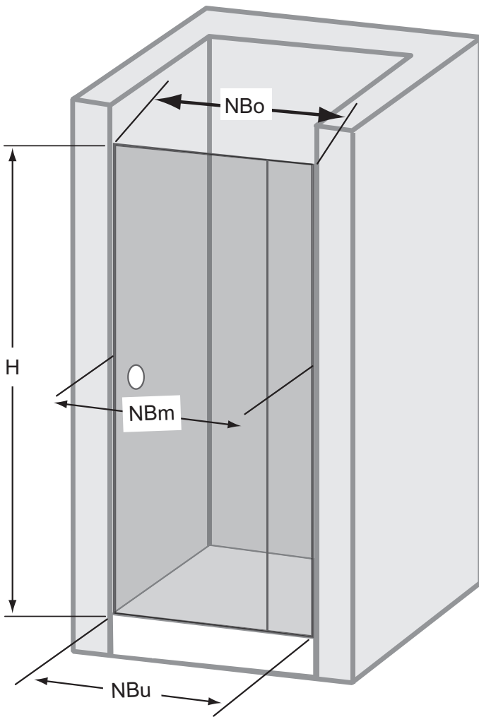
Nischentür Anschlag rechts - Sondermaß
