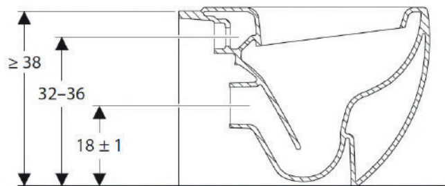
Abbildung 1: Anschlussbereiche/Auswahlkriterien für Stand-WC wandbündige Montage
