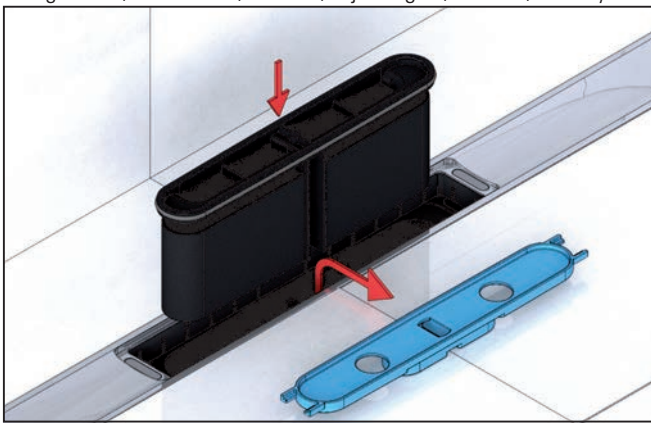
DallFlex / DallFlex Plan / CeraFlex / CeraFlex Plan waagrecht / horizontal / latéral / zijdelingse / lateral / bocznym
