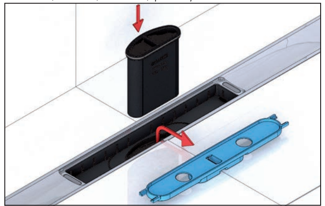
DallFlex / CeraFlex senkrecht / vertical / verticaal / pionowy
